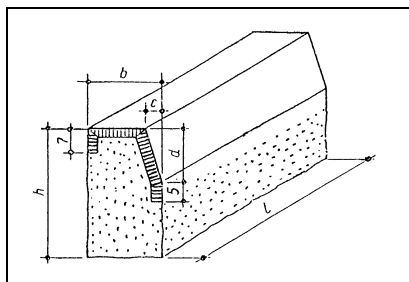
Rys. 2. Krawężnik uliczny odmiany UP, rodzaju B
